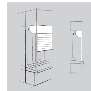
Pose sous linteau enroulement intérieur
