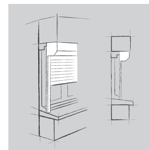
Pose sous linteau enroulement extérieur
